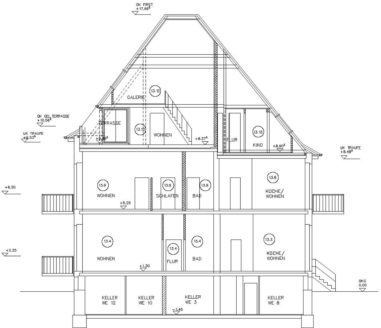
SNITT A - A
